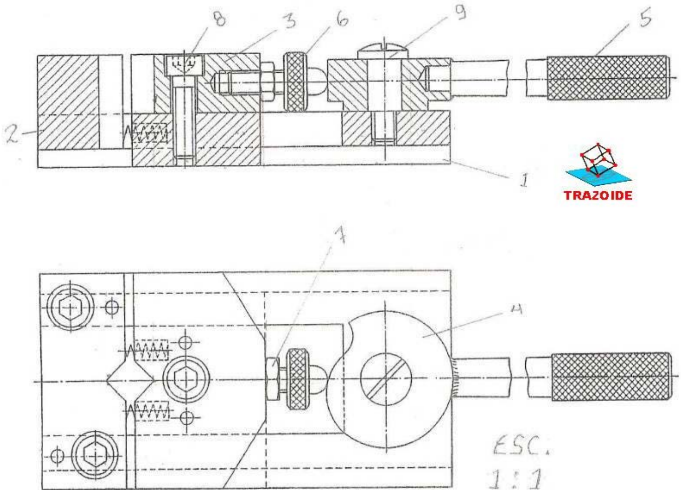
Fig. 17.10 Mordaza especial de ajuste rápido.
